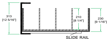
A-A VIEW
