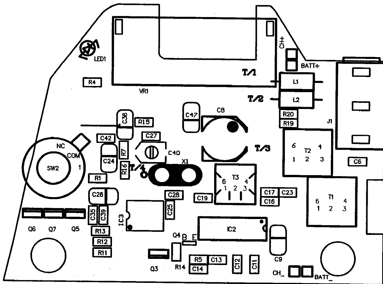
TopOverlay
