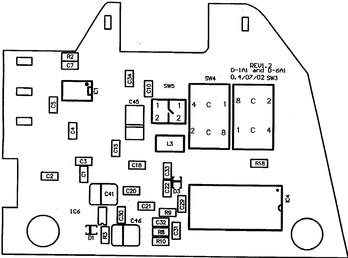
Bot Overlay
